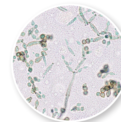
CLADOSPORIUM
